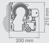
Stiprina pie sienas Wall installation Настенная установка
