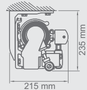
Stiprina pie griestiem Ceiling installation Потолочная установка
