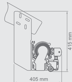
Stiprina pie spārēm Roof rafter installation Монтаж к кровли
